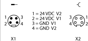
Napájecí konektor 7/8"
