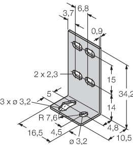
SMBQ12A 3074341 ángulo de montaje; material VA 1.4401, para optosensor modelo Q12
