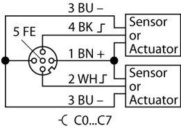
Złącze I/O M12 x 1
