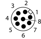
핀맵
