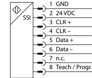
배선도
